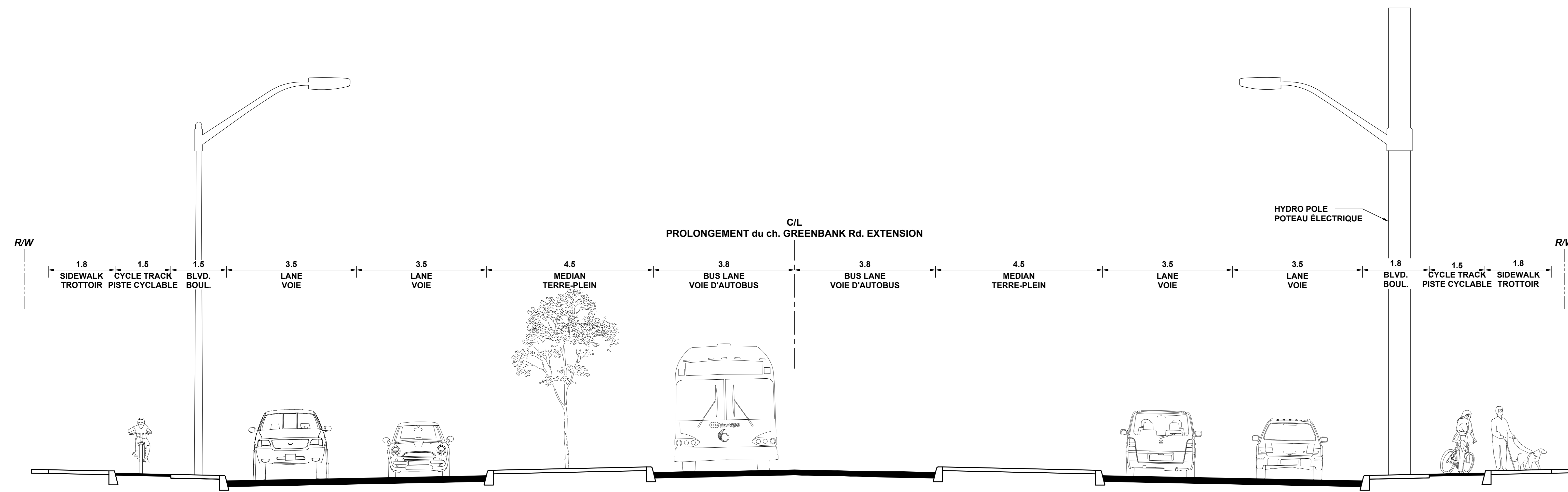
TYPICAL SECTION / TRONÇON TYPIQUE PROLONGEMENT du ch. GREENBANK Rd. EXTENSION 41.5m R/W N.T.S.
