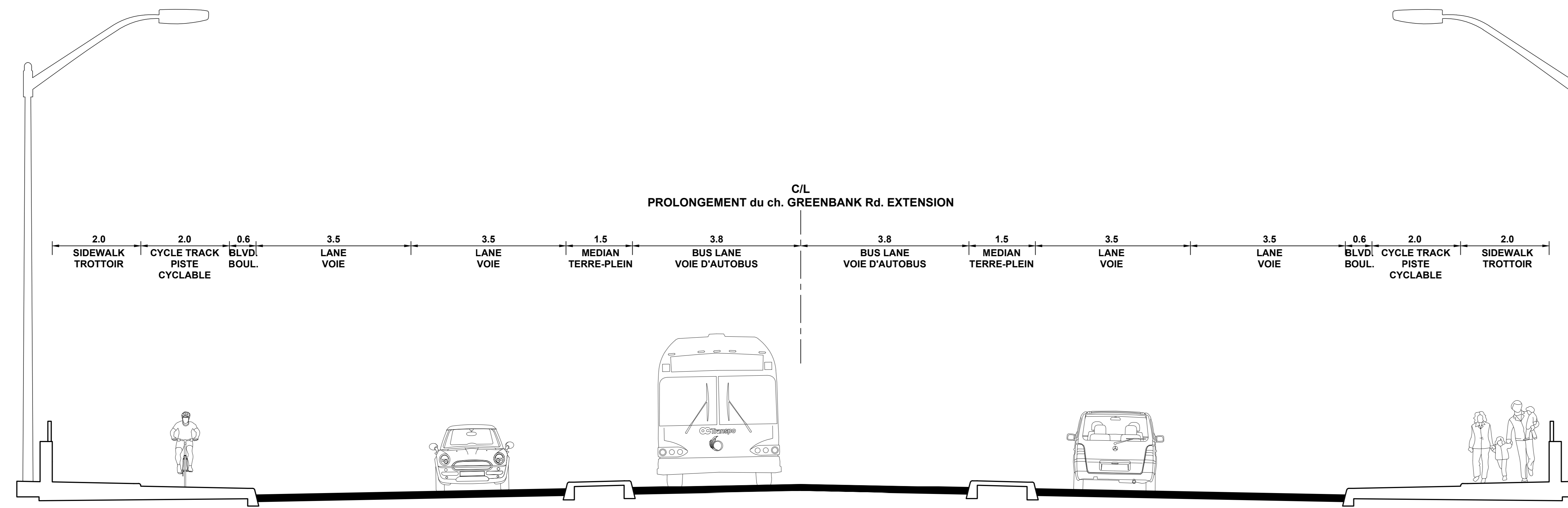
TYPICAL SECTION / TRONÇON TYPIQUE PROLONGEMENT du ch. GREENBANK Rd. EXTENSION BRIDGE / PONT N.T.S.
