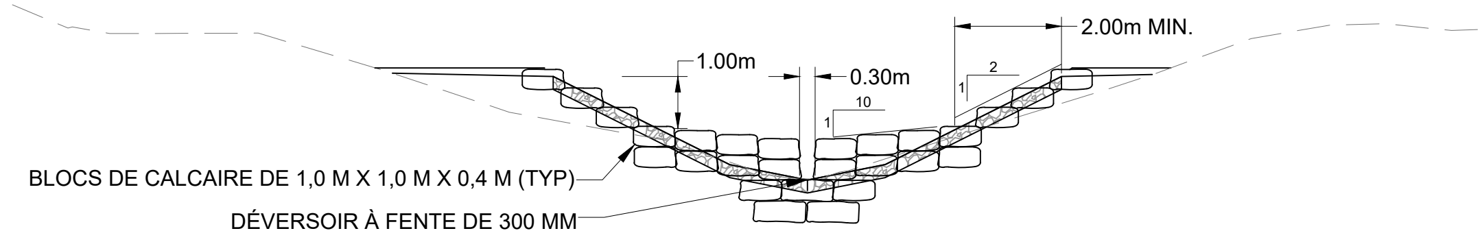
SECTION DU DÉVERSOIR A-A
