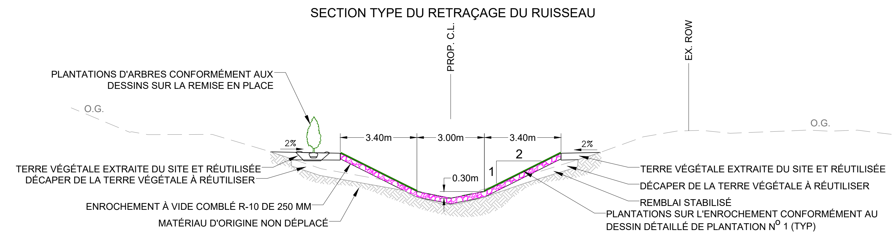
ZONE DE RÉPARATION N° 2 POUR LA STABILITÉ DES PENTES SECTION TYPE
