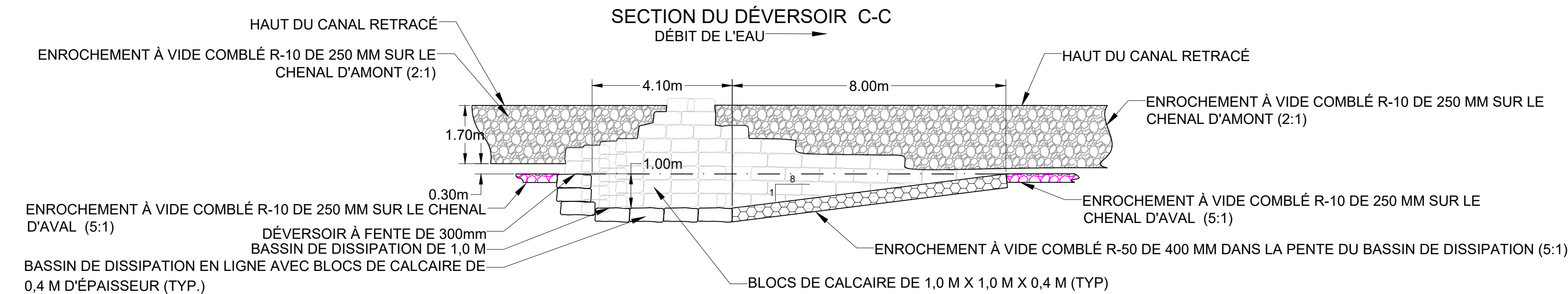
SECTION DU DÉVERSOIR C-C
