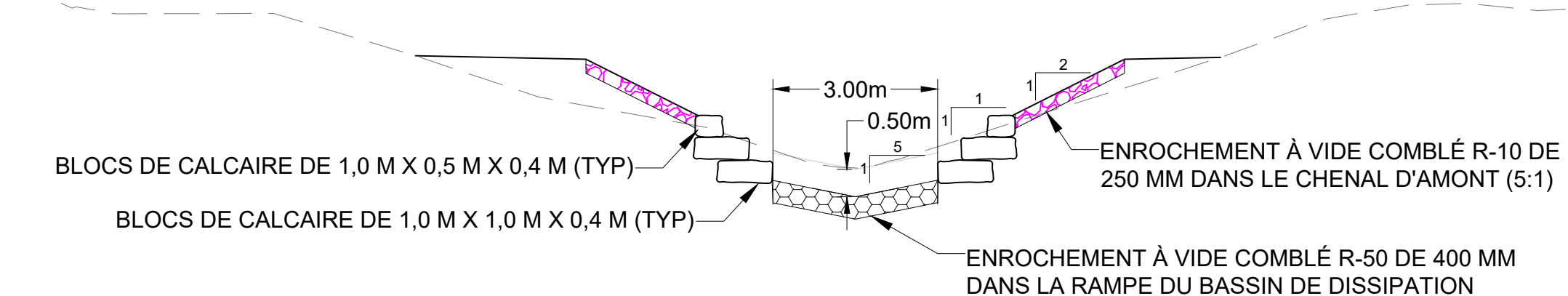
SECTION DU DÉVERSOIR B-B
