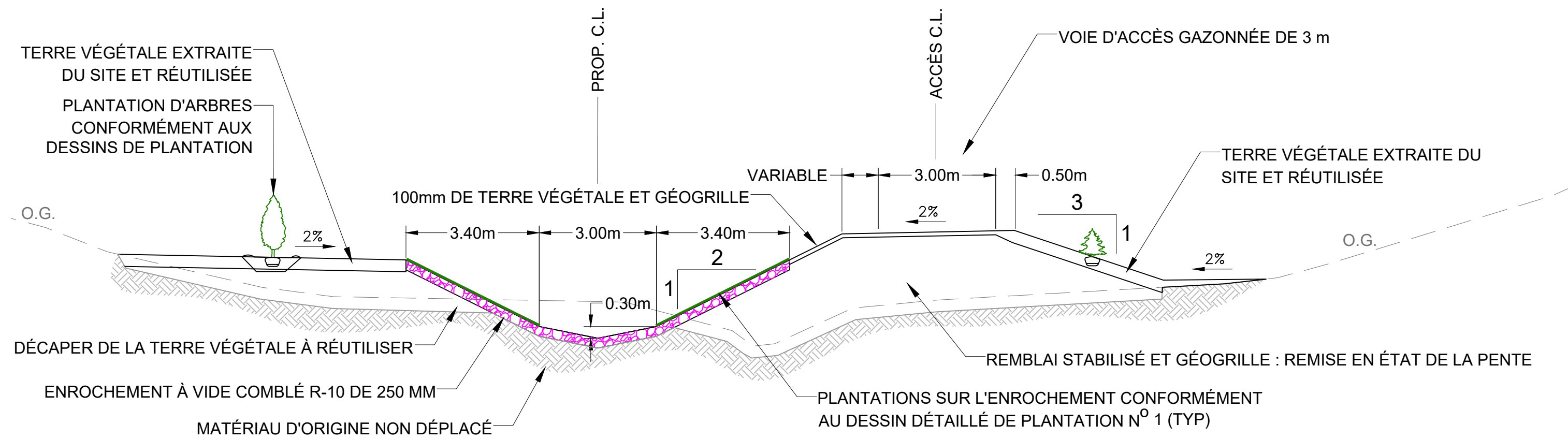
SECTION TYPE DU CHEMIN D'ACCÈS INFÉRIEUR
