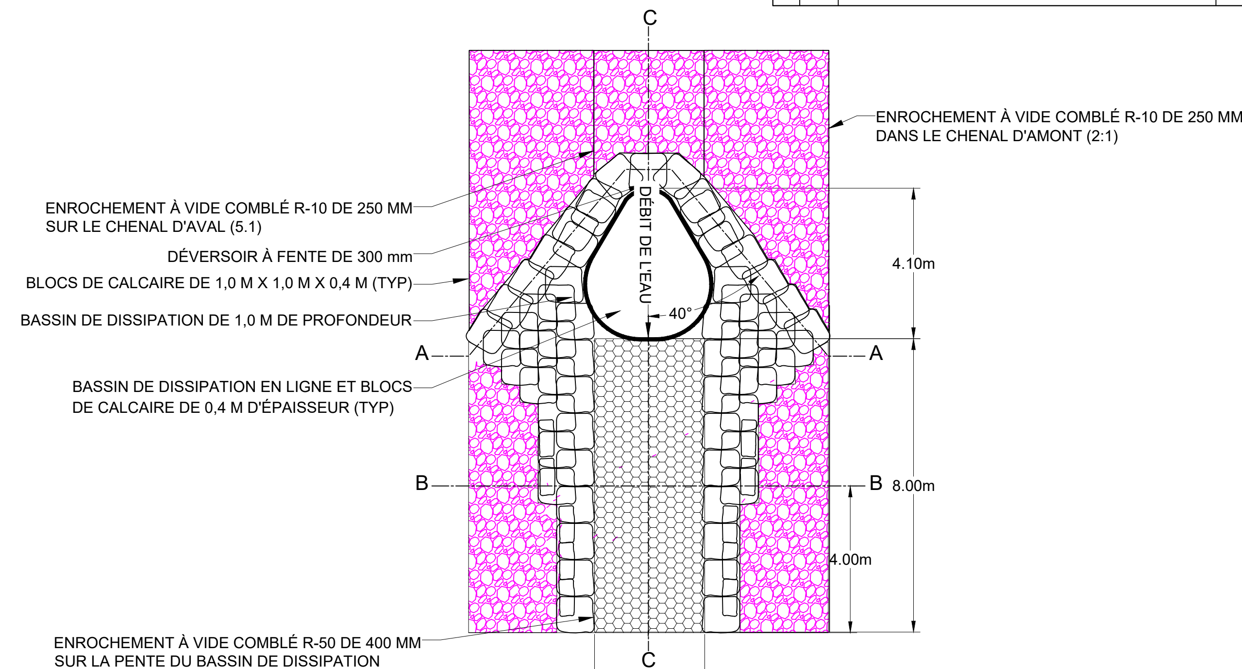
DÉTAIL DU DÉVERSOIR
