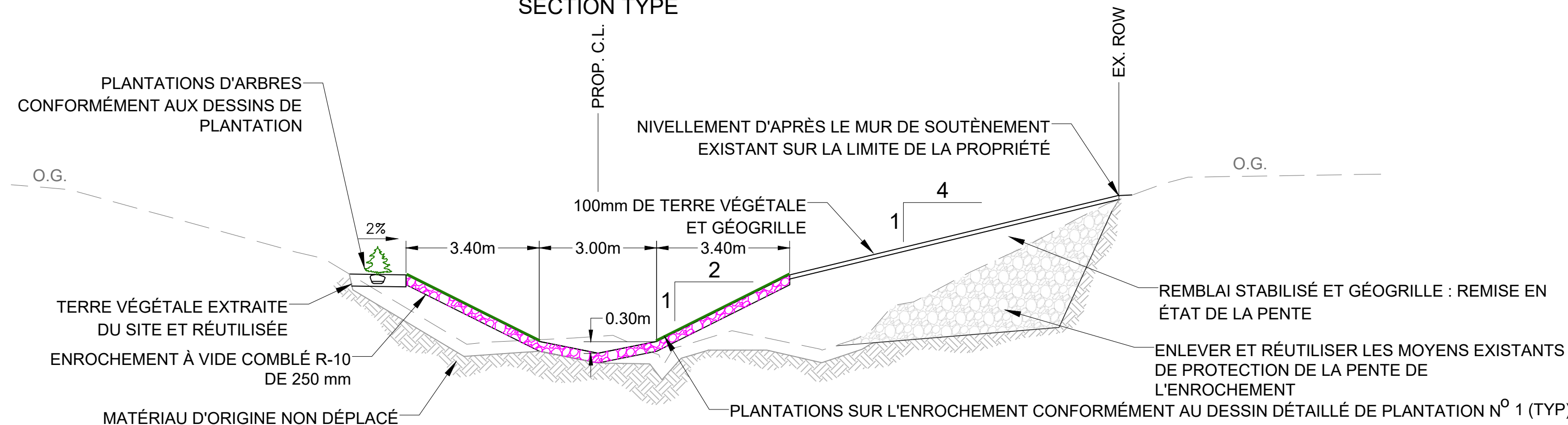
SECTION TYPE DU CHEMIN D'ACCÈS INFÉRIEUR
