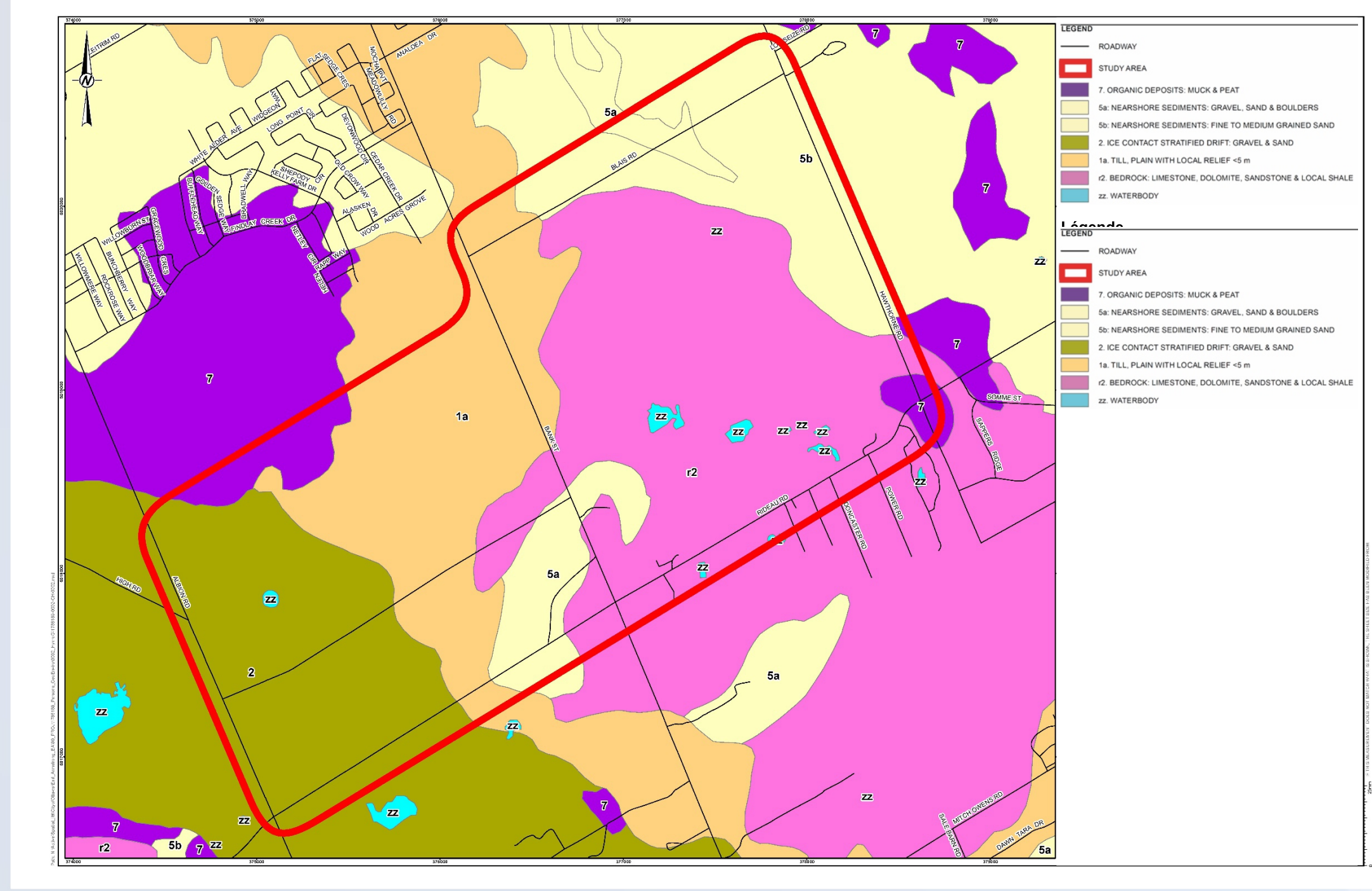
Surficial Geology Géologie des dépôts meubles
