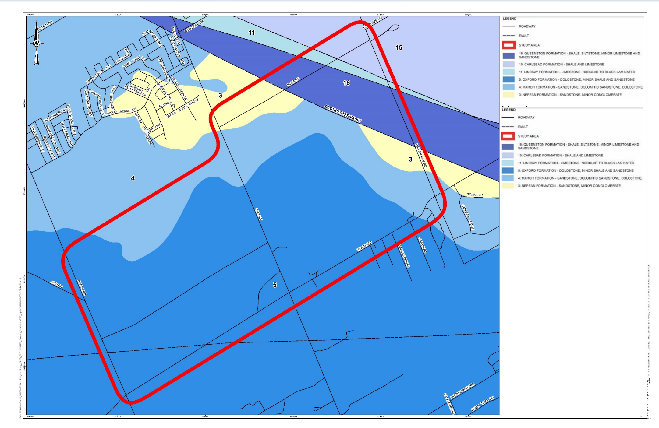
Bedrock Geology Géologie du soubassement
