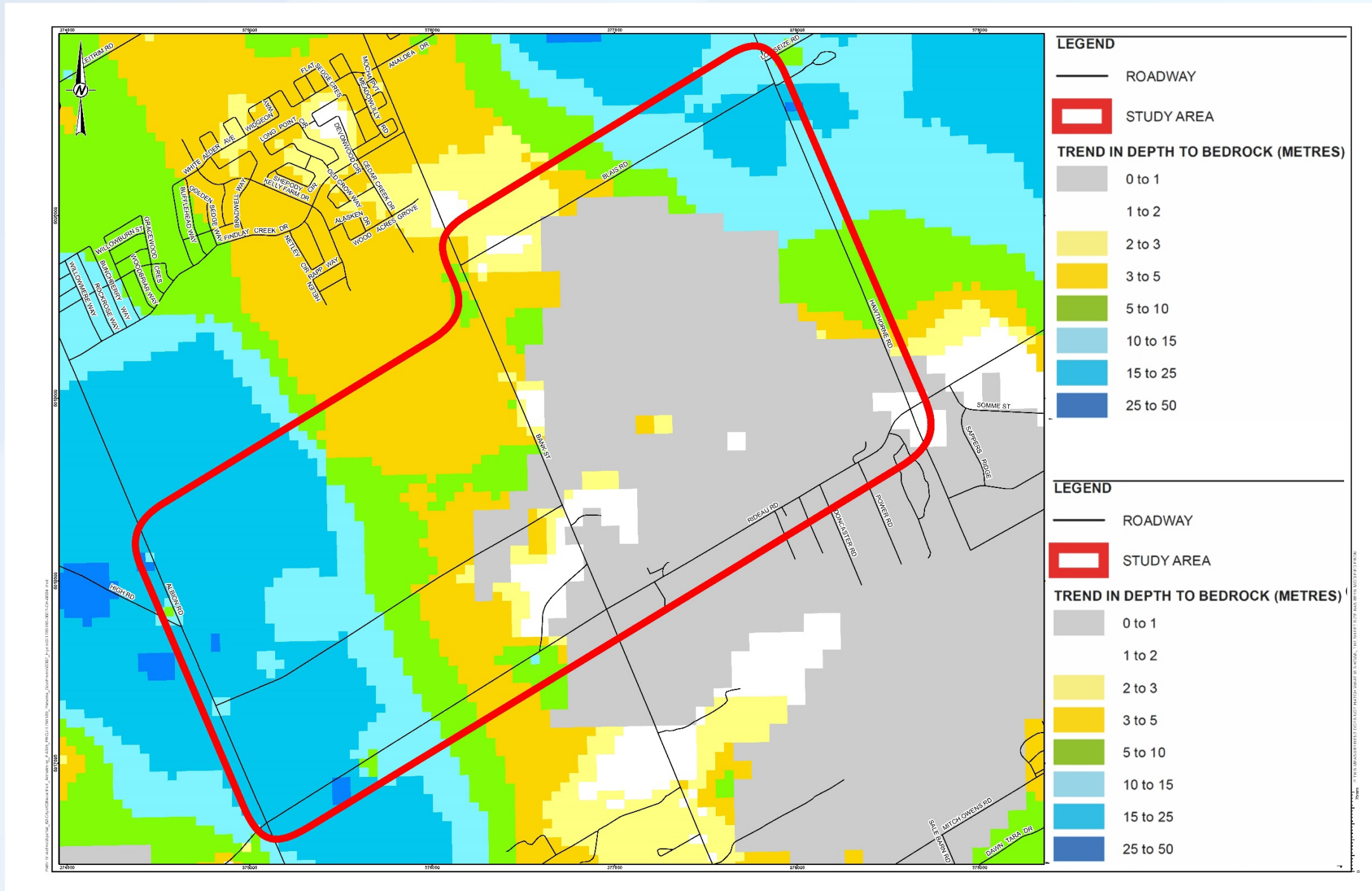
Drift Thickness Épaisseur de dérive
