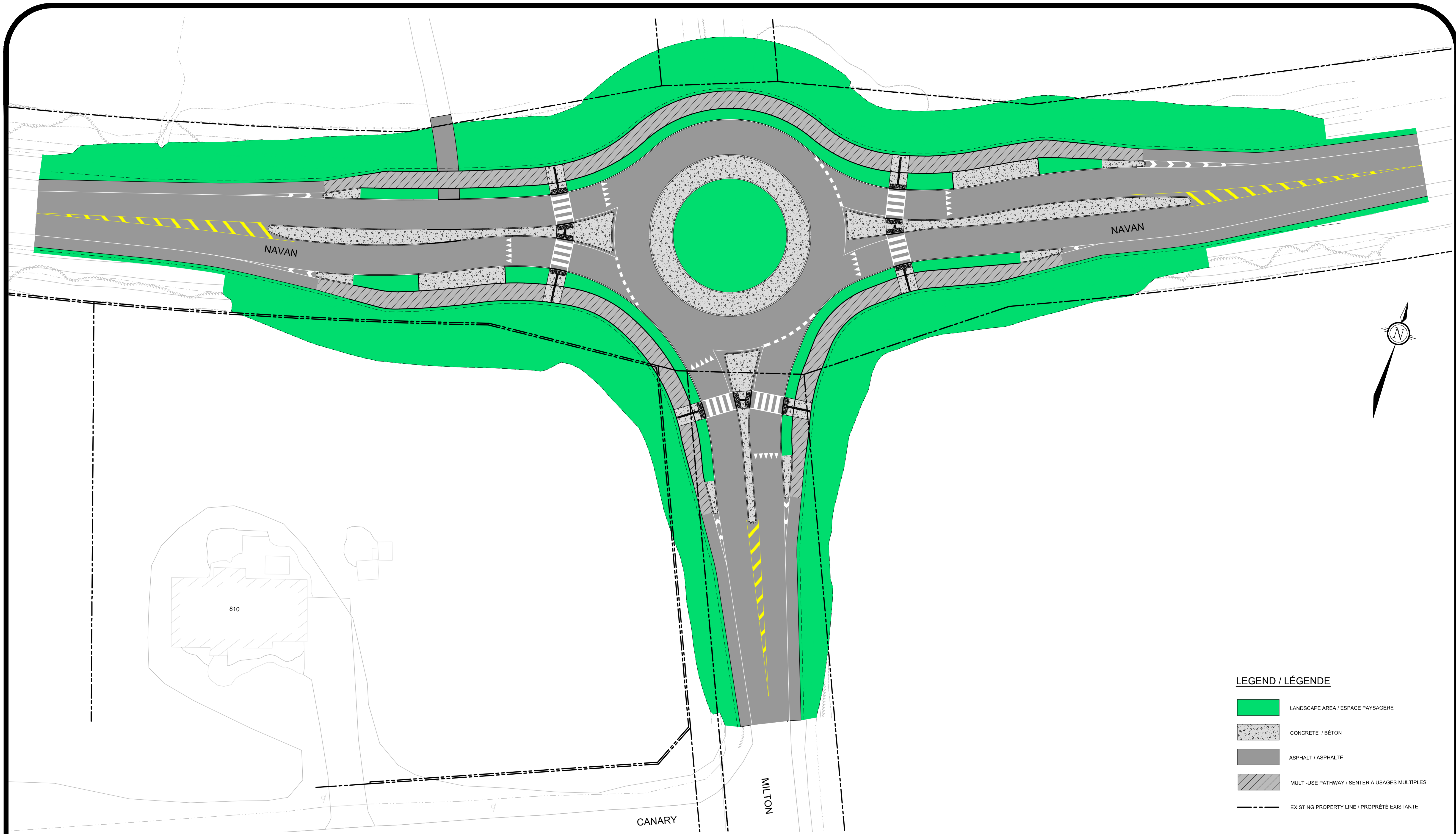
NAVAN ROAD AND MILTON ROAD DEVELOPMENT ROUNDABOUT - GEOMETRY / AMÉNAGEMENT D'UN CARREFOUR GIRATOIRE À L'ANGLE DES CHEMINS NAVAN ET MILTON - GÉOMÉTRIE
