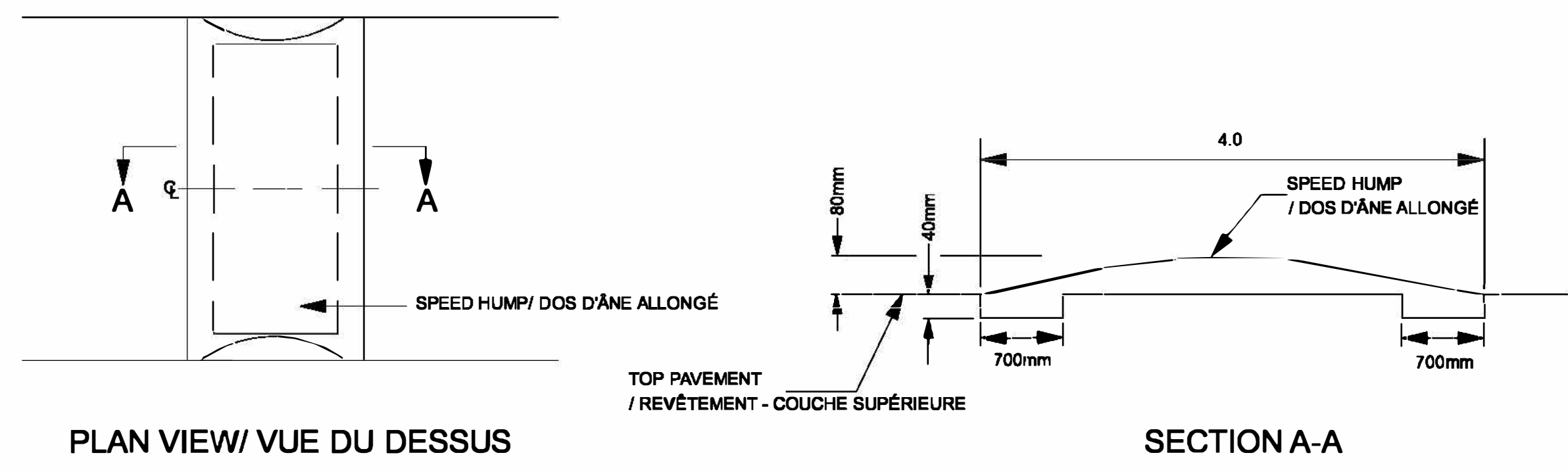
SPEED HUMP DETAIL/ DÉTAIL POUR LE DOS D'ÂNE ALLONGÉ
