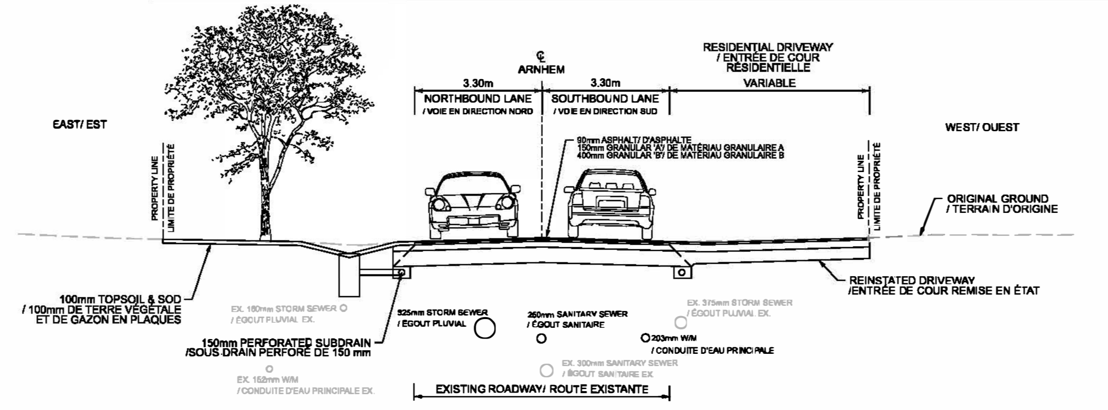
TYPICAL SECTION AT RESIDENTIAL DRIVEWAY /COUPE TRANSVERSALE TYPE - ENTRÉE DE COUR RÉSIDENNELLE
