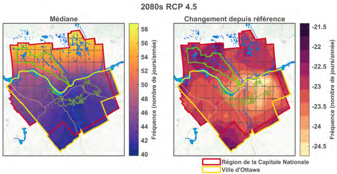
Figure F1.96: Nombre d'événements de gel profond (température minimale quotidienne < -10^{\circ}\text{C} ) - 2080s RCP 4.5.
