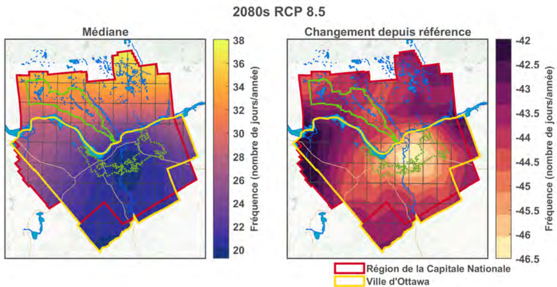
Figure F1.97: Nombre d'événements de gel profond (température minimale quotidienne < -10^{\circ}\text{C} ) - 2080s RCP 8.5.
