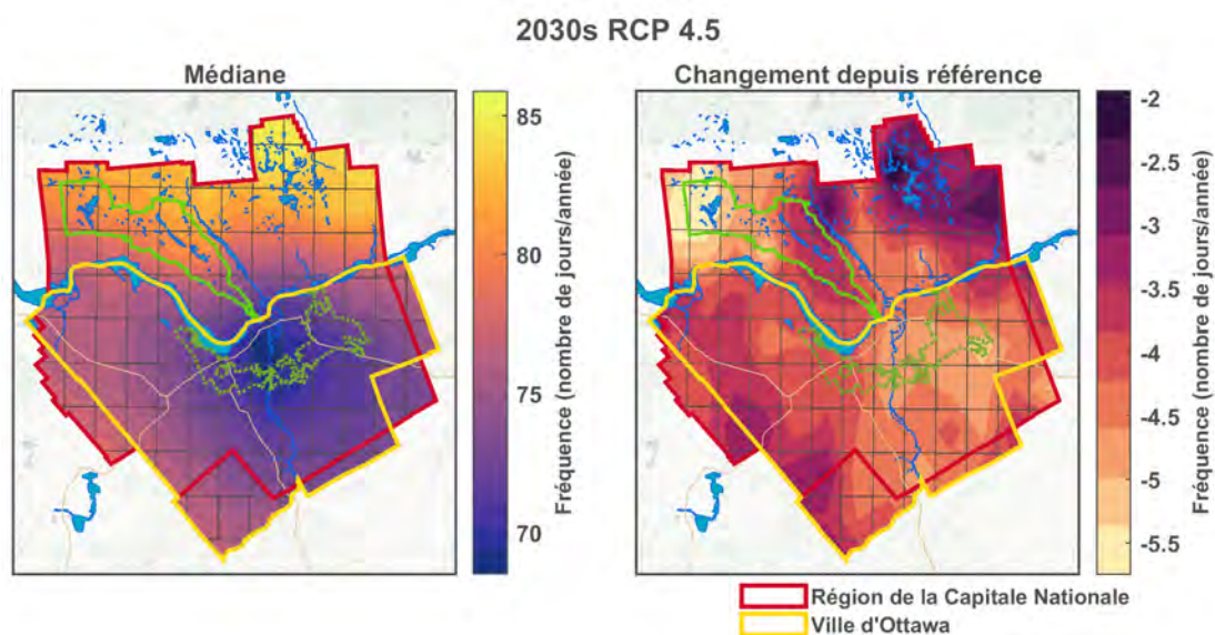
Figure F1.168: Cycles annuels de gel et de dégel - 2030s RCP 4.5.
