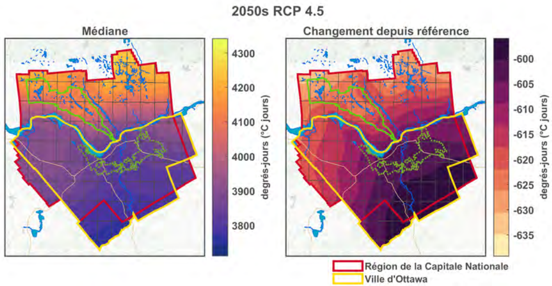
Figure F1.195: Degrés-jours de chauffage (18°C).
