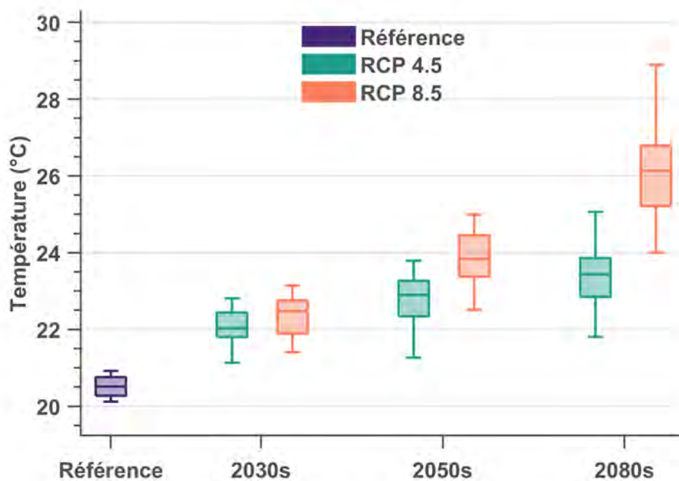
Figure F1.128: Température moyenne mensuelle - juillet.
