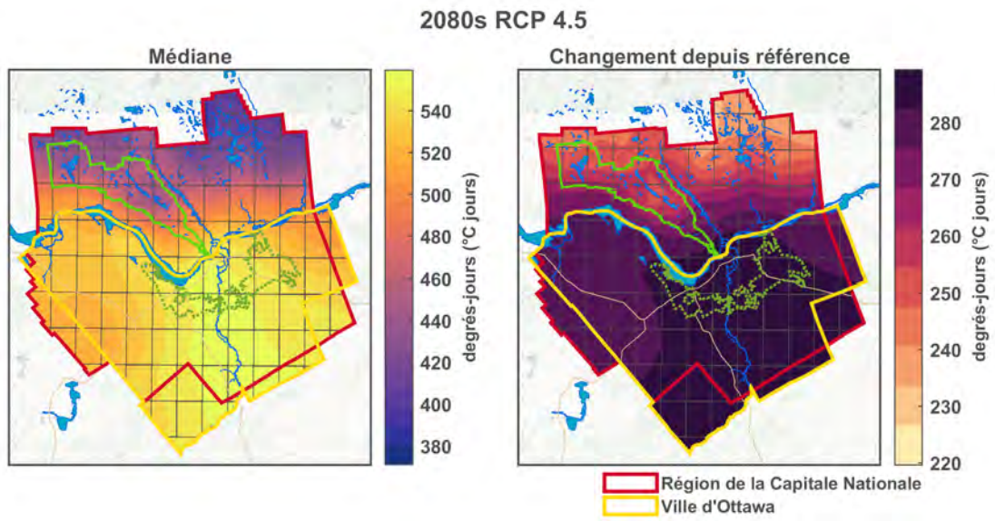
Figure F1.207: Degrés-jours de refroidissement (18°C) - 2080s RCP 4.5.
