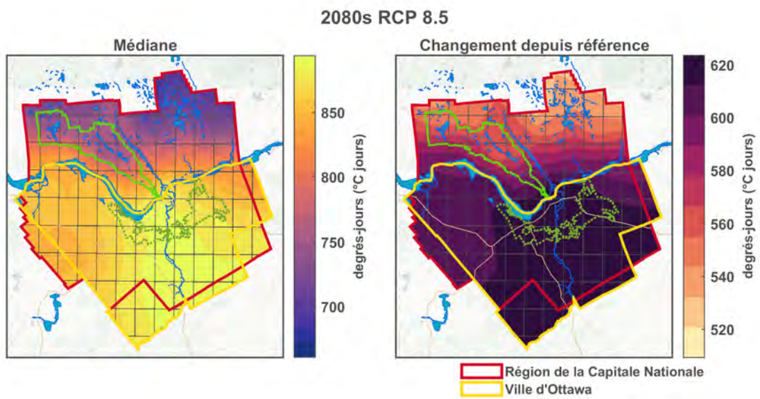
Figure F1.208: Degrés-jours de refroidissement (18°C) - 2080s RCP 8.5.
