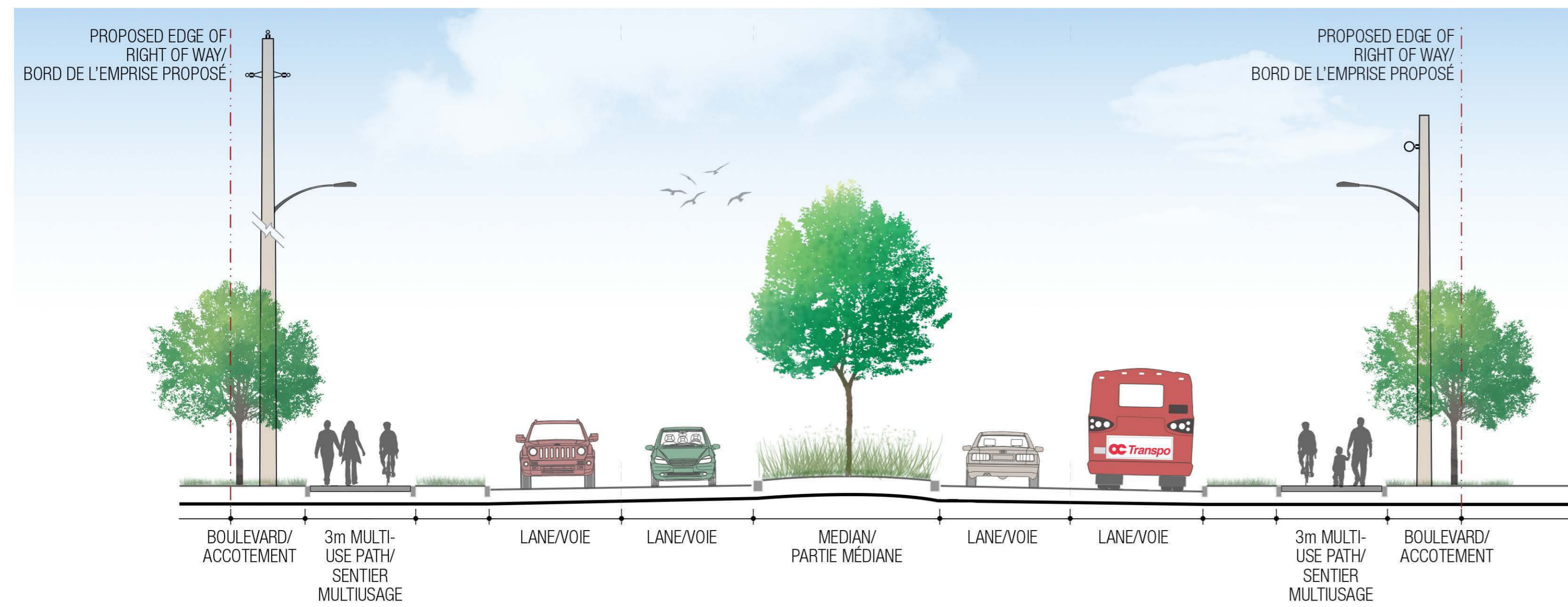
SECTION A-A
