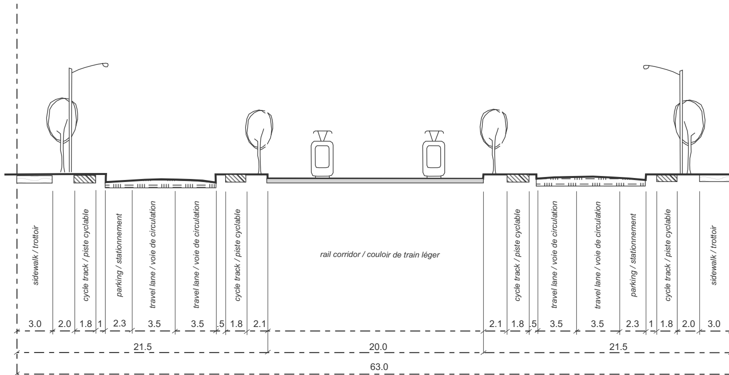
APPENDICE 3 RIVERSIDE-SUD - CENTRE COUPE TRANSVERSALE DE LA « RUE DU TRANSPORT EN COMMUN » (à l'est du chemin Limebank)
