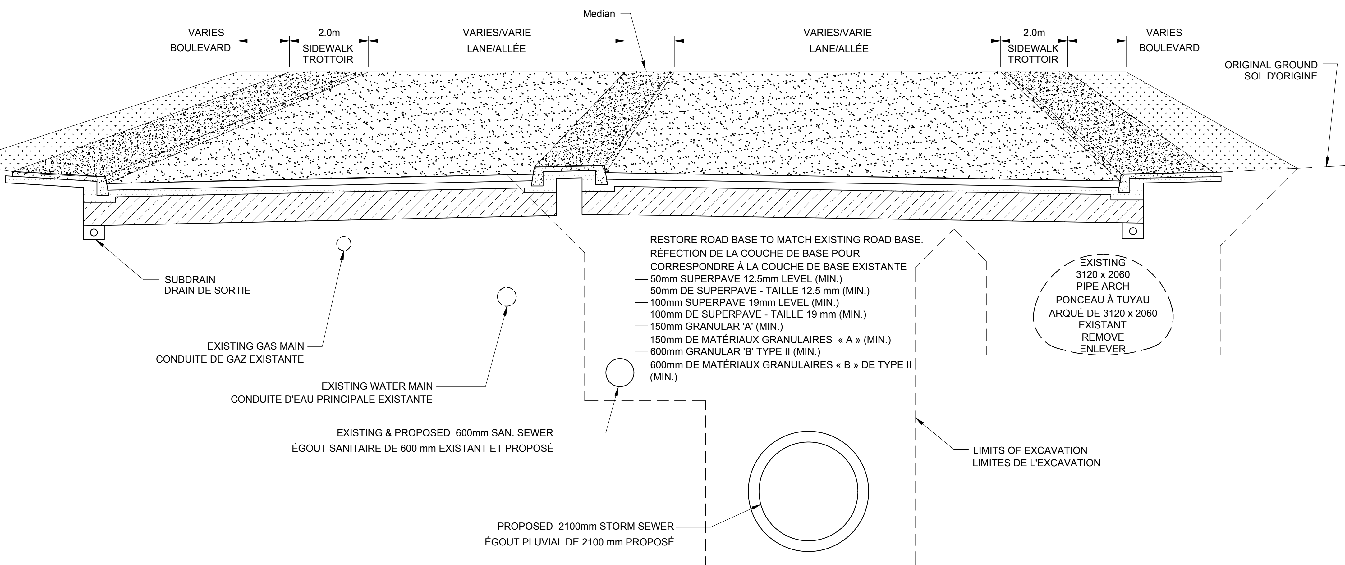
ST. LAURENT BOULEVARD MEDIAN SECTION/SECTION MÉDIANE DU BOULEVARD ST-LAURENT
