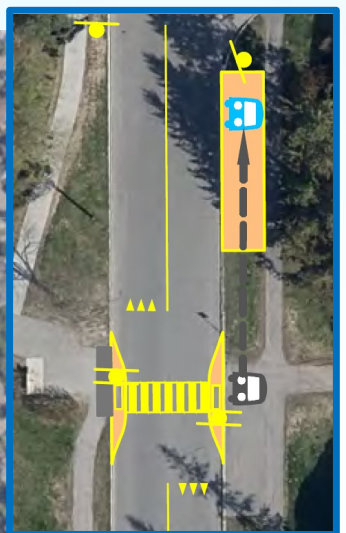
Passage pour piétons avec avancées de trottoir et déménagement de l'arrêt de bus
