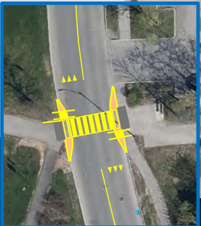
Passage pour piétons avec avancées de trottoir
