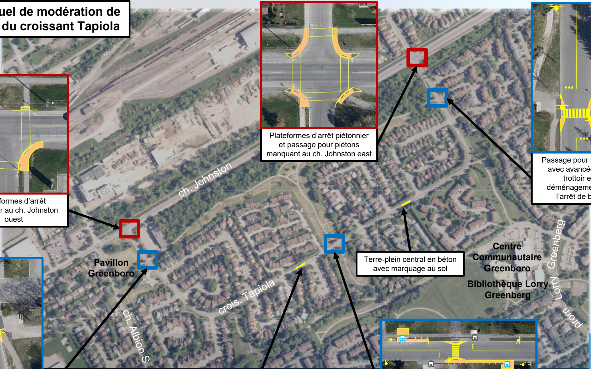
Terre-plein central en béton avec marquage au sol
