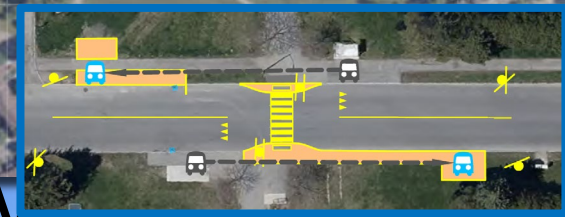
Passage pour piétons avec avancées de trottoir et déménagement des arrêts de bus
